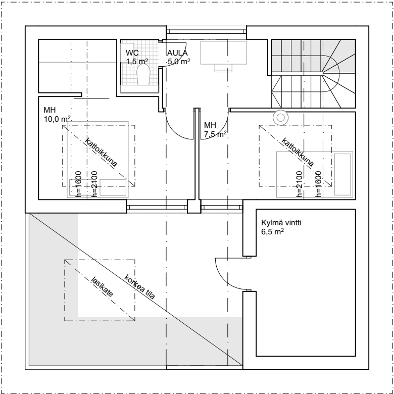
2.krs
