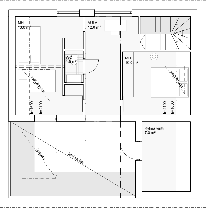
2.krs
